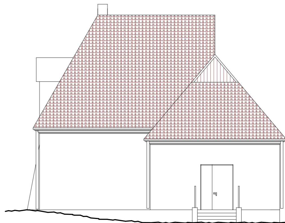
ELEWACJA PÓŁNOCNA
